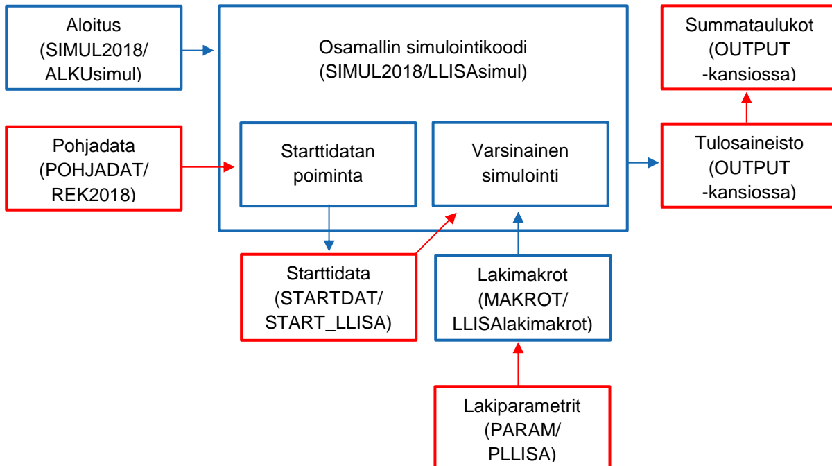
Kuva 1. Osamallin simulointiohjelman kulku. Esimerkkinä lapsilisämalli (LLISA). Siniset laatikot ovat SAS-koodia ja punaiset laatikot SAS-aineistoja. Summataulukot tulostuvat sekä SAS-aineistoiksi, että SAS-ohjelman sisäiseen tulosikkunaan. Halutessaan ne voi myös tallentaa automaattisesti Excel-tiedostoiksi.
