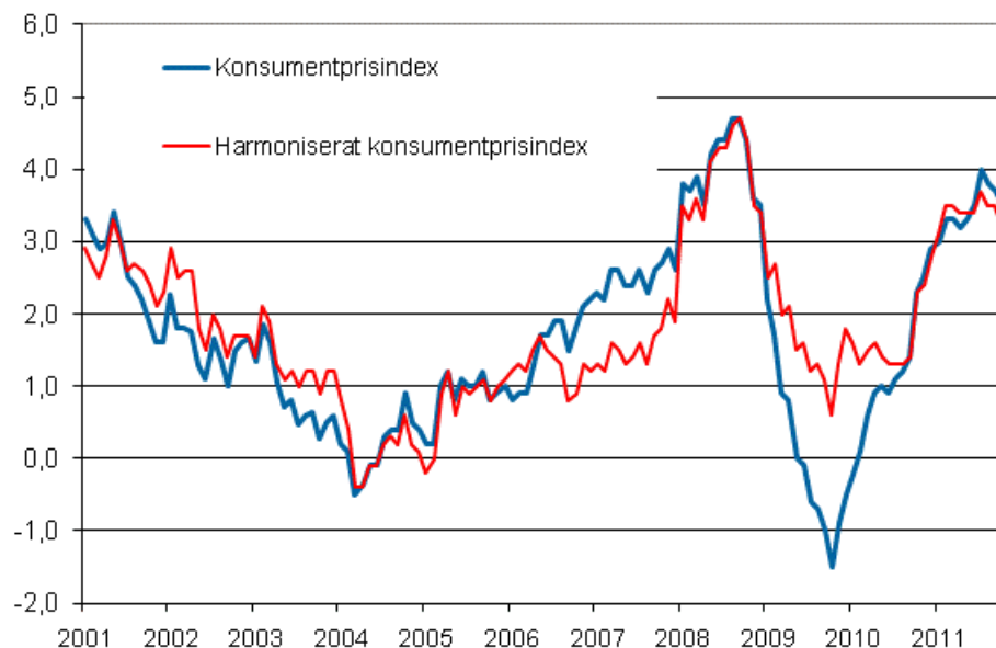
Figurbilaga 1. Årsförändring av konsumentprisindexet och det harmoniserade konsumentprisindexet, januari 2001 - oktober 2011
