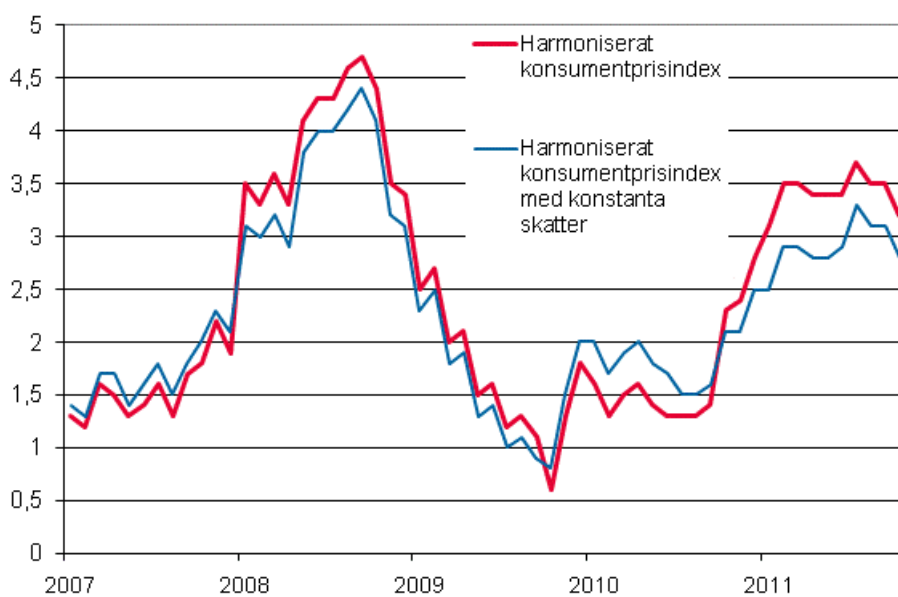
Figurbilaga 3. Årsförändring av det harmoniserade konsumentprisindexet och det harmoniserade konsumentprisindexet med konstanta skatter, januari 2007 - oktober 2011
