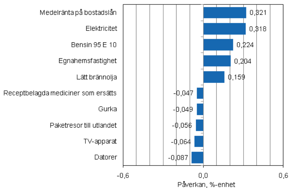
Figurbilaga 2. Varor och tjänster som har mest påverkat årsförändringen av konsumentprisindexet i oktober 2011
