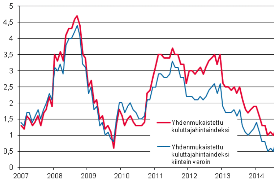
Liitekuvio 3. Yhdenmukaistetun kuluttajahintaindeksin ja yhdenmukaistetun kuluttajahintaindeksin kiintein veroin vuosimuutokset, tammikuu 2007 - elokuu 2014
