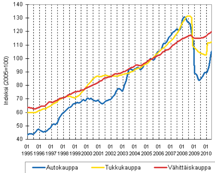
Liitekuvio 1. Auto-, tukku- ja vähittäiskaupan liikevaihdon trendisarjat (TOL 2008)
