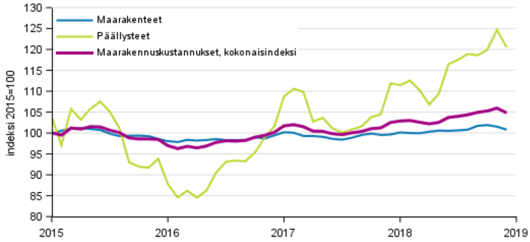
Liitekuvio 1. Maarakennusindeksin (2015=100) kokonaisindeksin, maarakennetöiden ja päällysteiden kustannuskehitys 1/2015–12/2018
