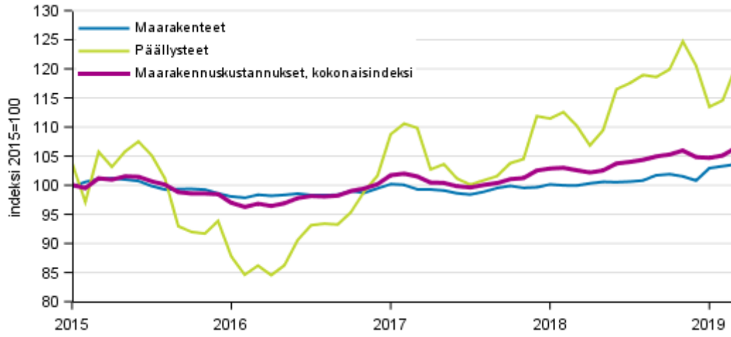
Liitekuvio 1. Maarakennusindeksin (2015=100) kokonaisindeksin, maarakennetöiden ja päällysteiden kustannuskehitys 1/2015–3/2019
