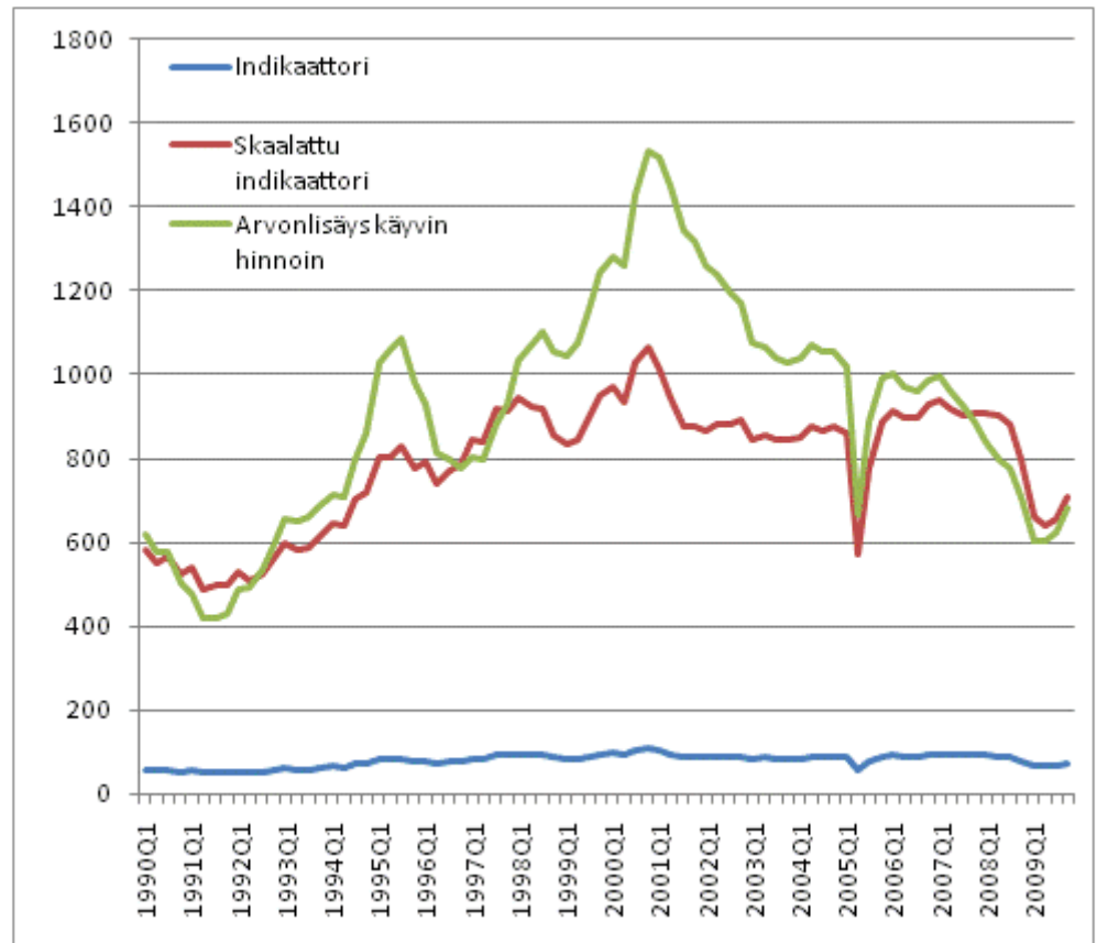
Kuva 1: Indikaattori ja suhteellisella Denton-menetelmällä täsmäytetty aikasarja
