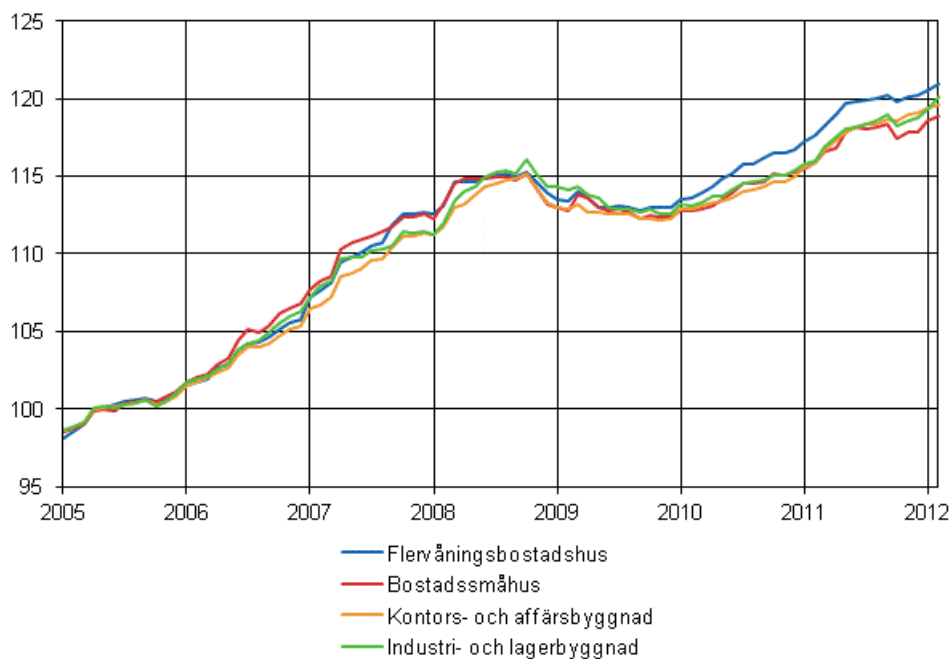
Figurbilaga 1. Byggnadskostnadsindex 2005=100
