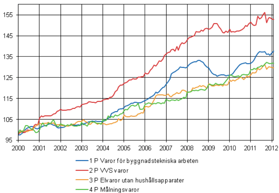
Figurbilaga 2. Indexvillkor-delindex 2000=100
