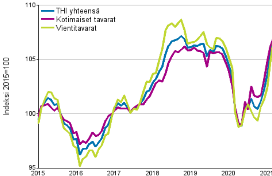
Tuottajahintaindeksi (THI) 2015=100, 1/2015–03/2021
