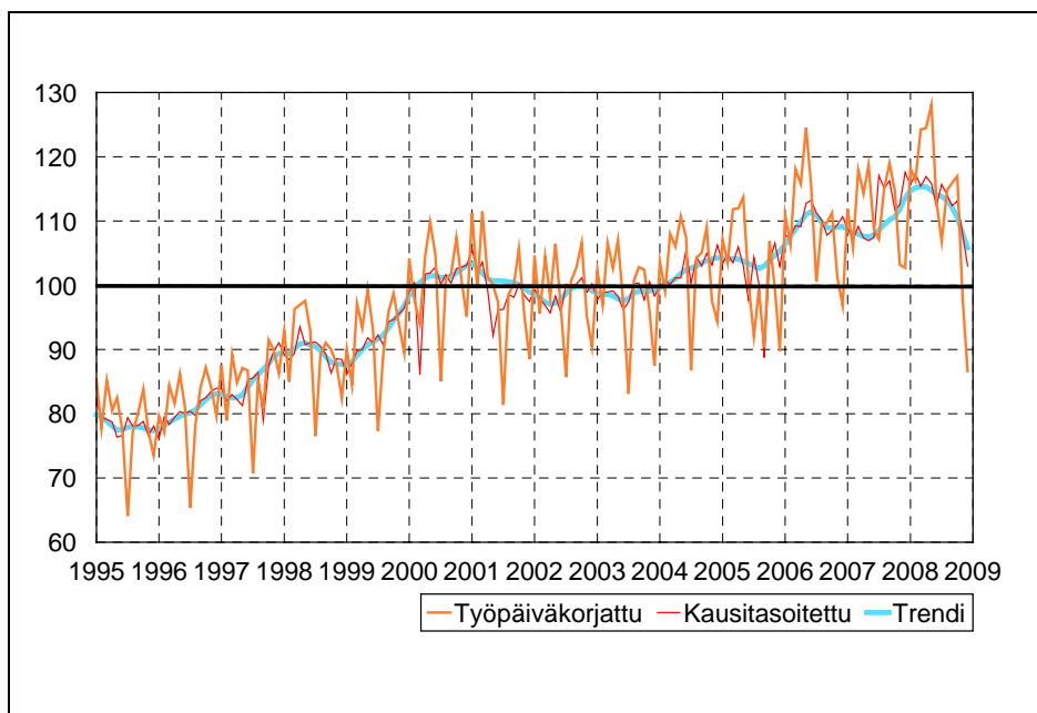
Kuvio 8. Kemianteollisuus TOL 23-25, teollisuustuotannon volyyymi-indeksi 1995 – 2008 joulukuu, 2000=100
