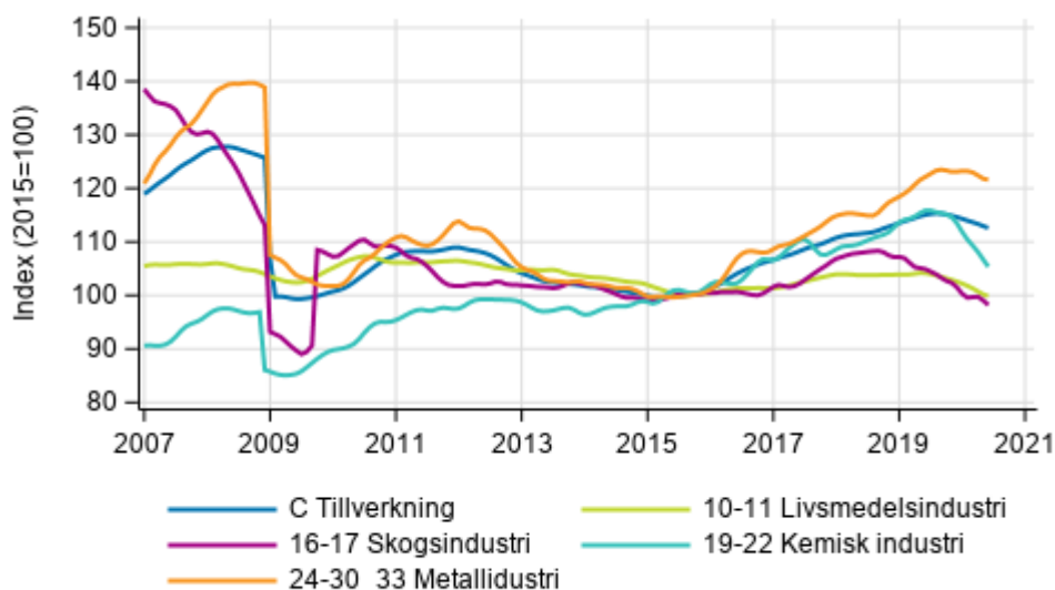
Figurbilaga 2. Trendserien för undernäringsgrenar inom industriproduktionen 2007/01– 2020/05, TOL 2008
